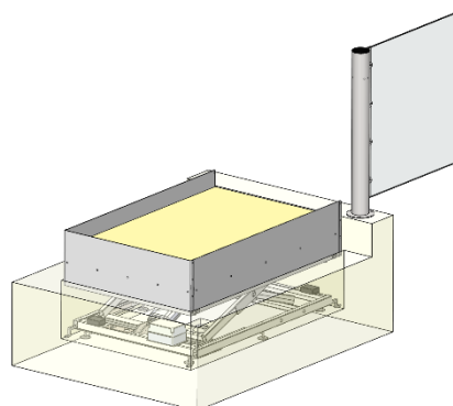
Niveau supérieur
